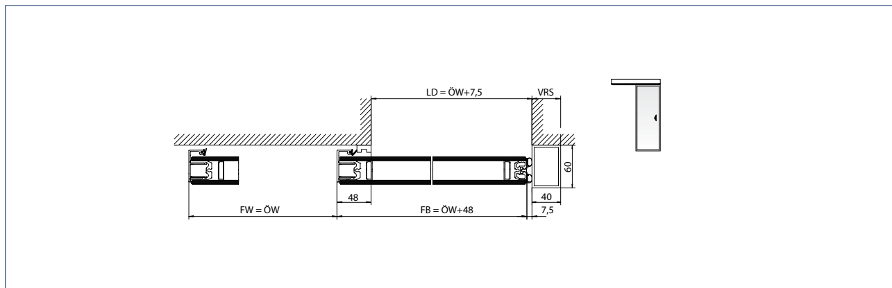
1-křídlový dveřní systém LD = Světlý průchod FW = Dráha
