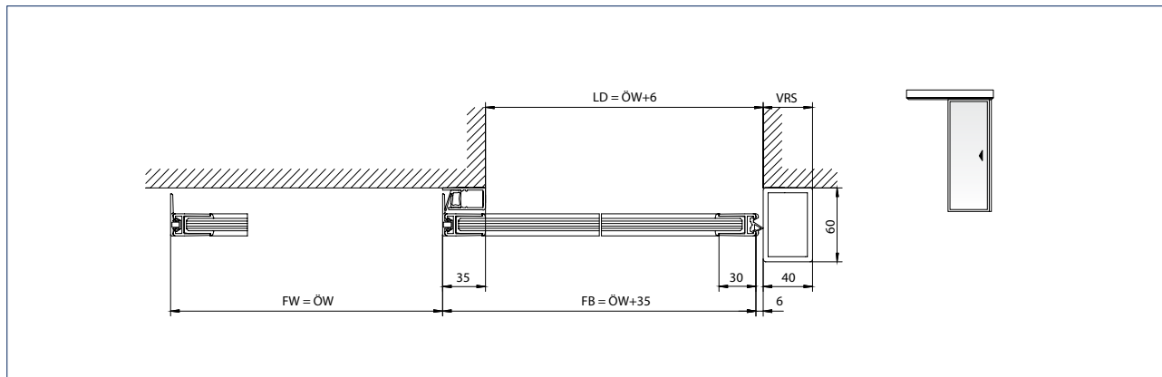
1-křídlový dveřní systém LD = Světlý průchod FW = Dráha FB = Šířka křídla ÖW = Šířka otevření VRS = Prodloužení pohonu vpravo
